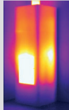
3 hod. od zatopení Průměrná teplota povrchu 88 °C
